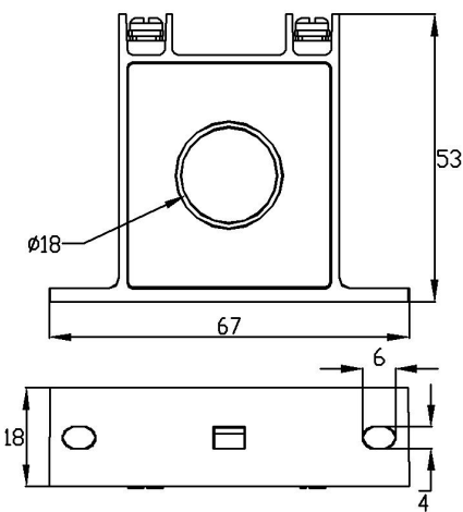
互感器尺寸图（尺寸单位 mm）
