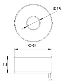
互感器尺寸图（尺寸单位 mm）
