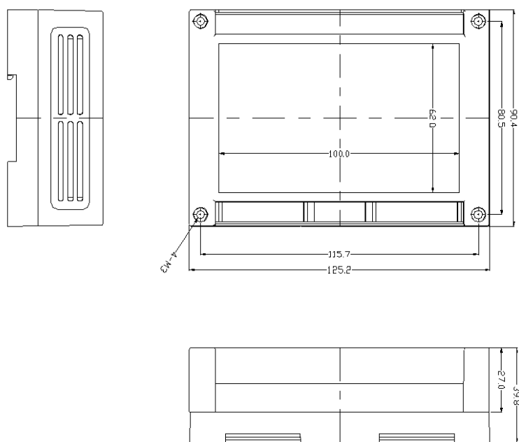
控制器尺寸图（尺寸单位 mm）备注：通过 DIN35 标准导轨安装
