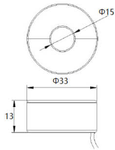
互感器尺寸图（尺寸单位 mm）线长 1m
